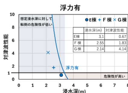
図6 3階建RC造建築物の転倒に対する対津波性能
