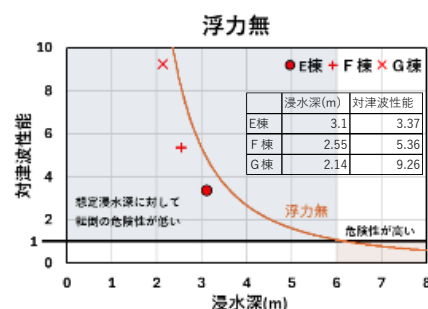
図6 3階建RC造建築物の転倒に対する対津波性能
