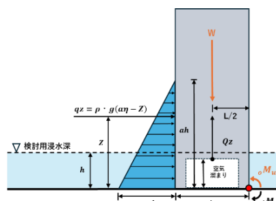
図5 津波波力と転倒の想定
