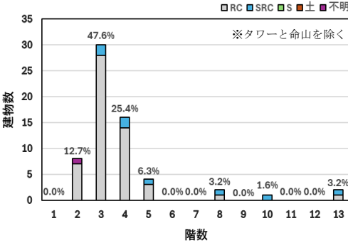
図2 避難施設の階数分布
