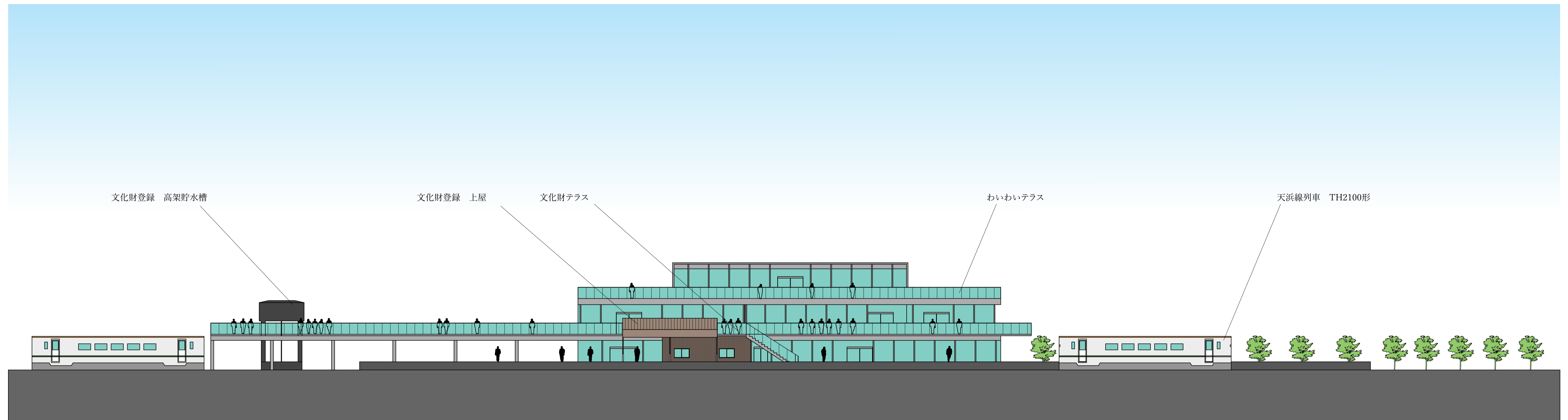
南立面図 1/200
