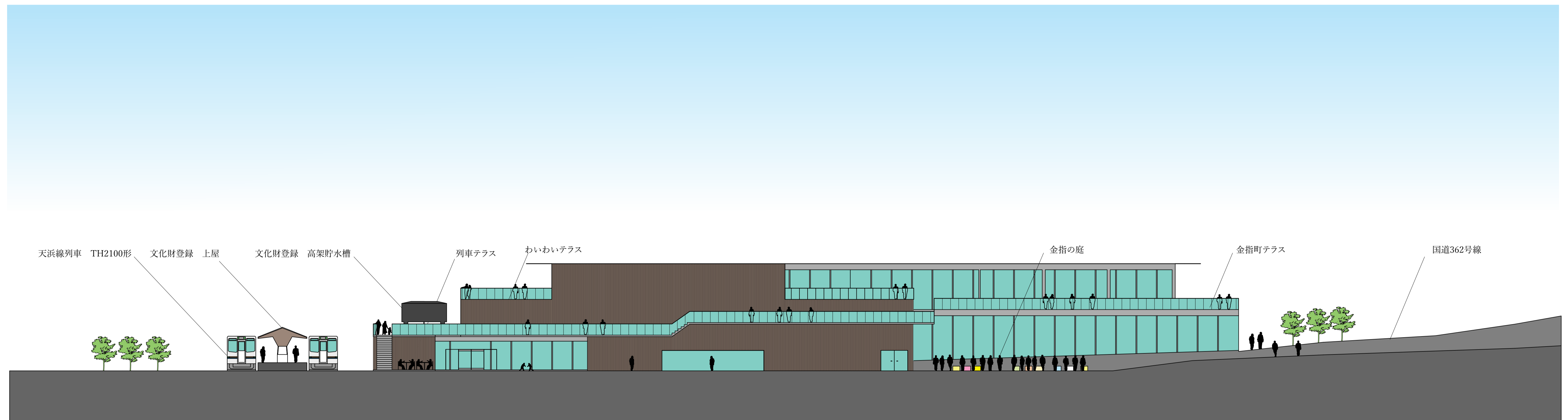
東立面図 1/200
